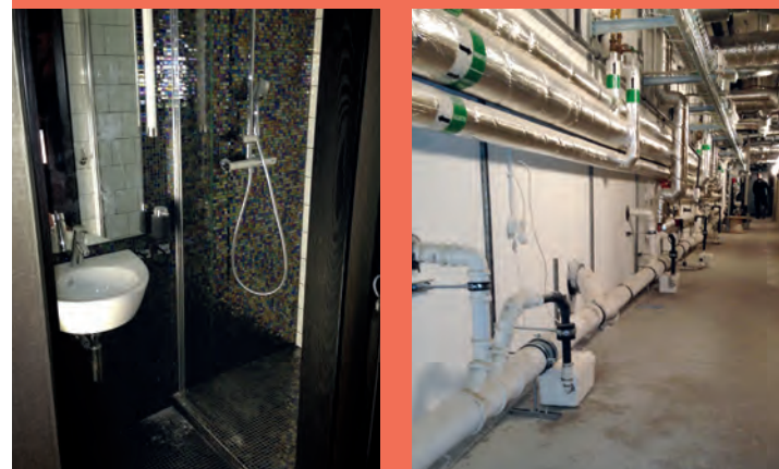
SANISHOWER® Flat instalovaný v technickém prostoru za koupelnou
